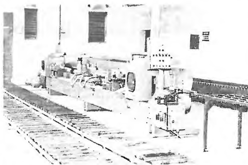
Novi stroj za postforming v TP Stari trg
