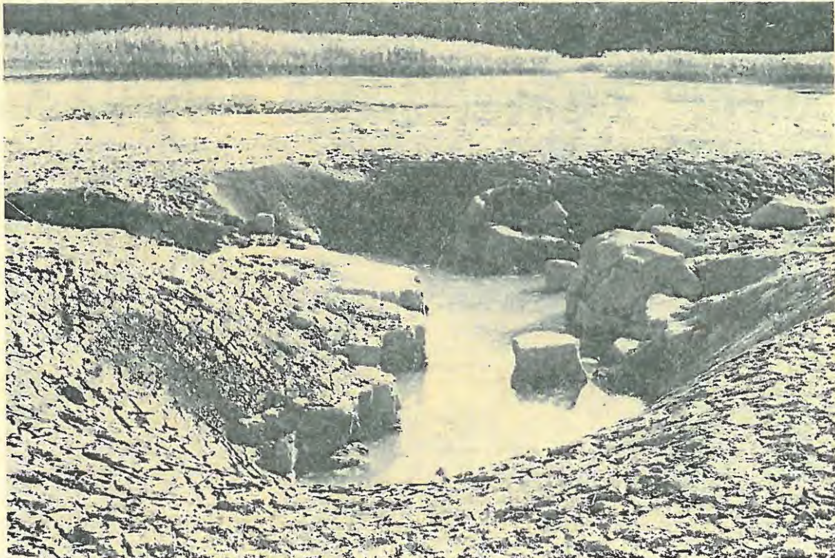
Avgustovsko usihanje Cerkniškega jezera
