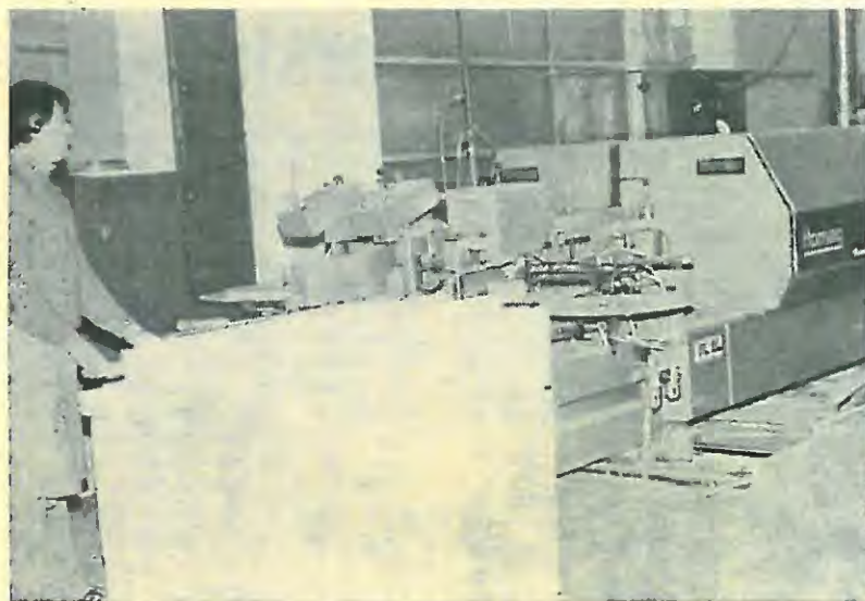
Novi stroj za furniranje robov
