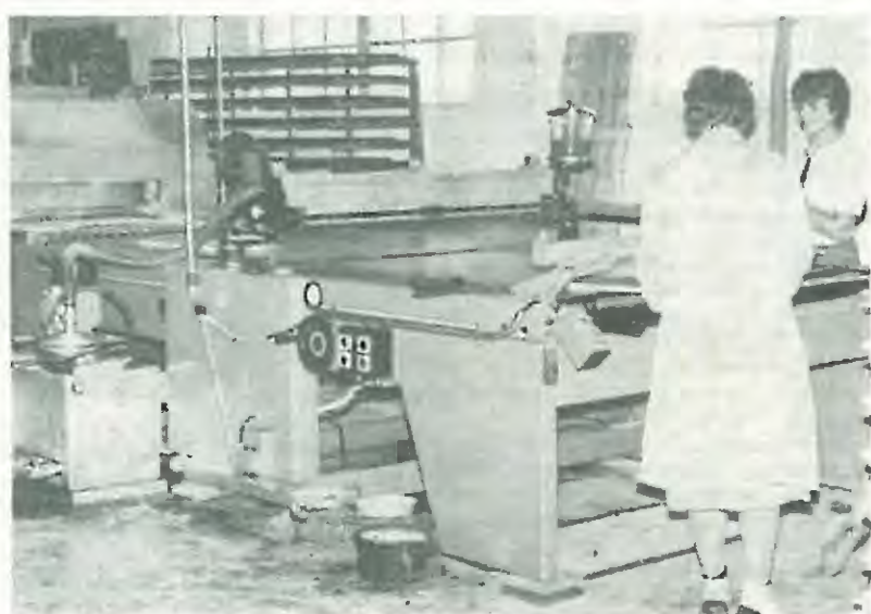
Polivalka laka (iz Brestove strojegradnje) na »poskusnem delu« v JELKI
