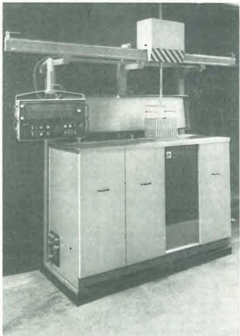
Iz Tozda Strojegradnje — Programirana naprava za ultrazvočno čiščenje kovinskih delov, ki jo izdelujejo v kooperaciji z Inštitutom za elektronsko in vakumsko tehniko iz Ljubljane.
