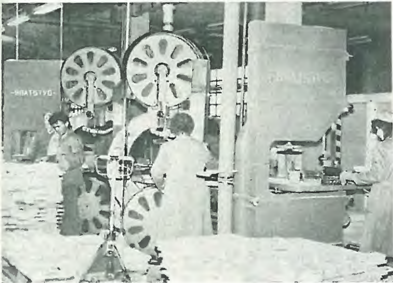
Razrez na tračnih žagah
