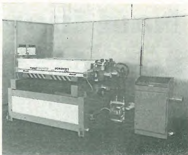
Valjna nanašalka laka: stroj, izdelan v sodelovanju s firmo Sorbini, od katerega si v Tozdu Strojgradnja veliko obetajo.
